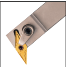
MVUN□95°
