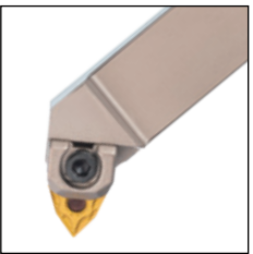
WWLN□95°
